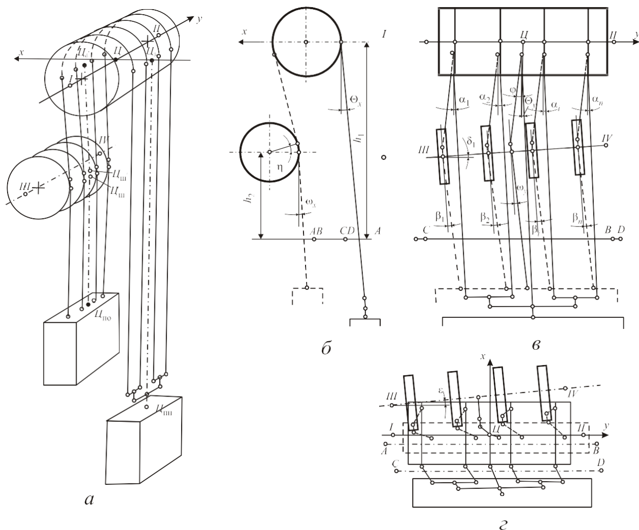
Рисунок 1. Геометричні елементи багатоканатної підйомної установки
