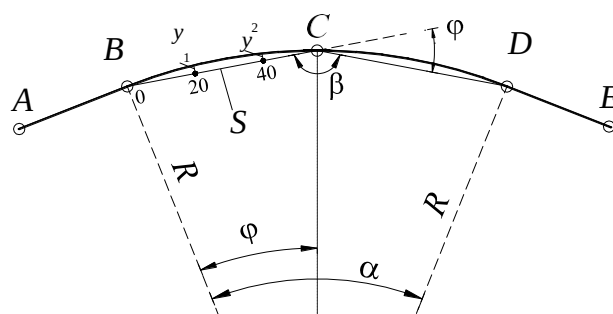
Рисунок 2. Зйомка кругової кривої у спосіб хорд
