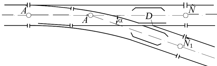
Рисунок 3. Розбивка стрілочного переходу
