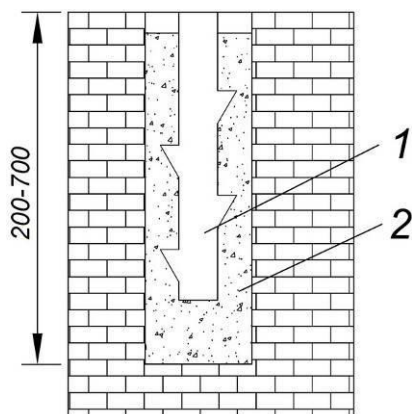
1 – металевий штир; 2 – бетон
